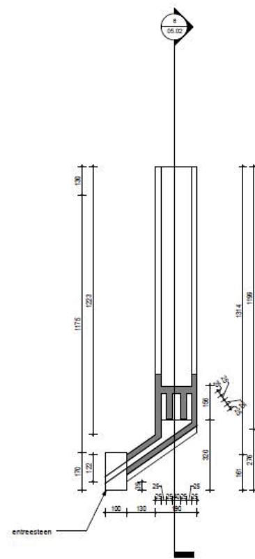
7 Drsn. 3 1:10
