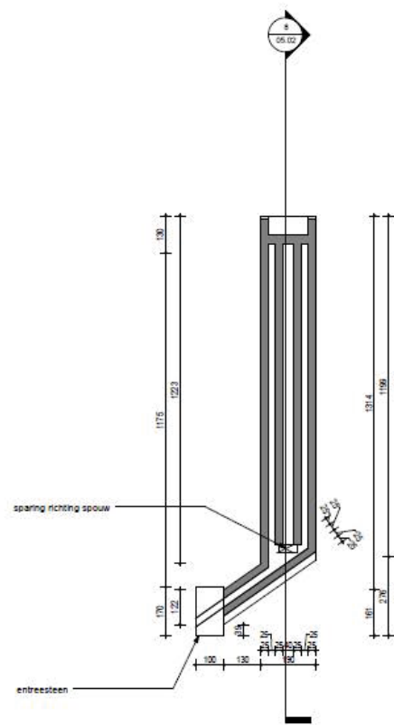
6 Drsn. 1 1:10
